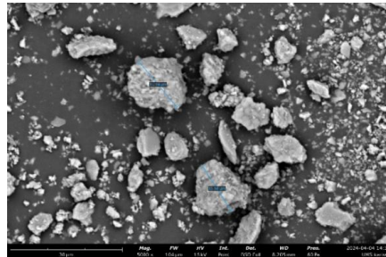
Gambar 1. Hasil uji SEM serbuk cangkang kerang hiaju perbesaran 5000x
