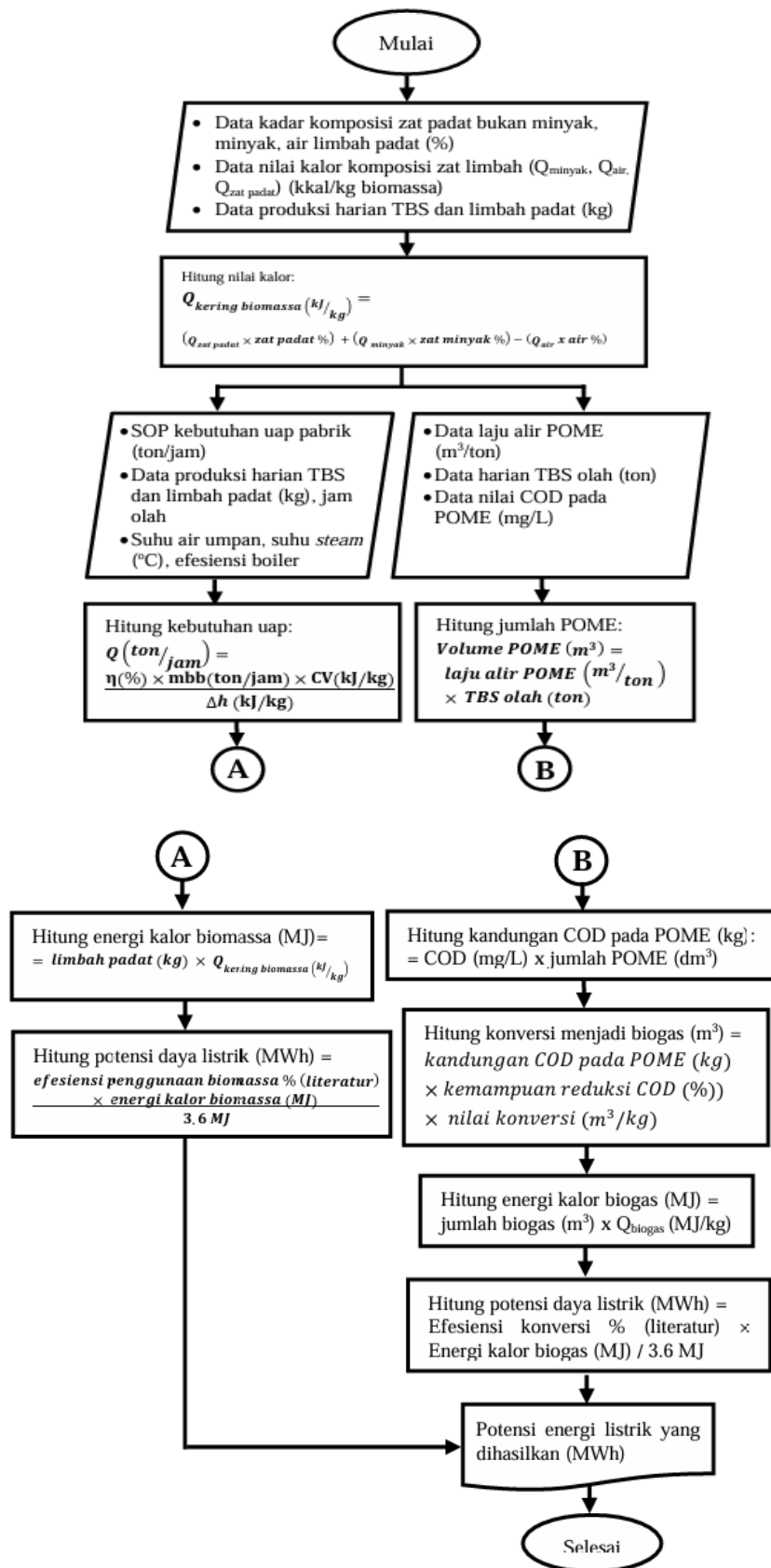
Gambar 1. Diagram alir analisis potensi limbah
